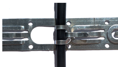
Крепление резистивного кабеля
