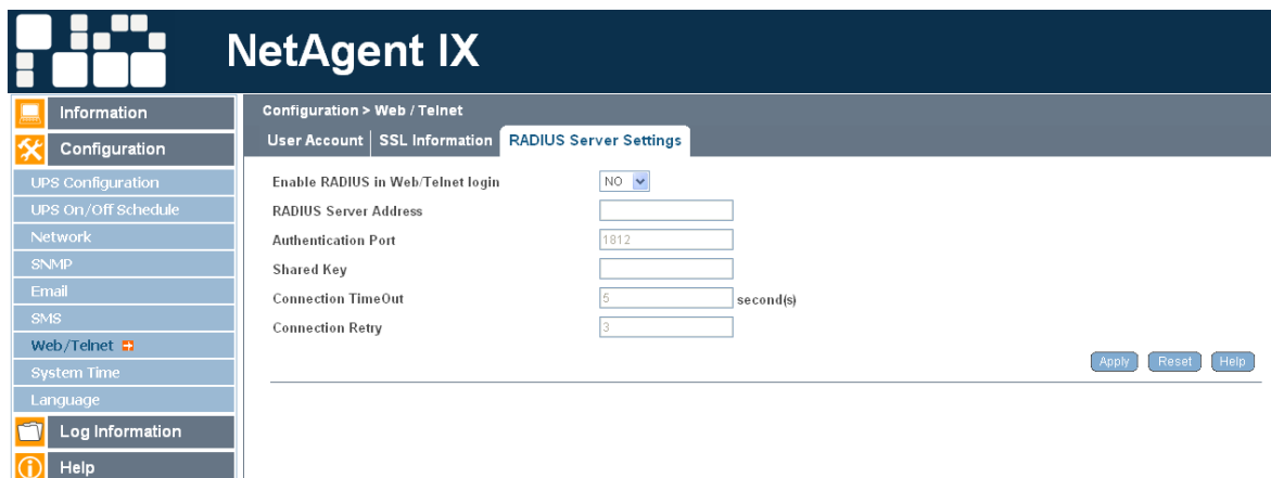
Рис.45 NetAgent 9 Radius
