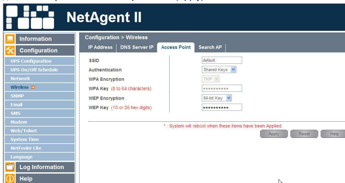
Рис 31. NetAgent 9 Беспроводная сеть
